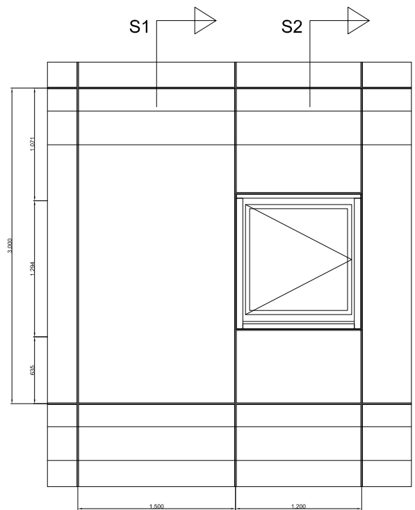
Alzado con modulo opaco y ventana
